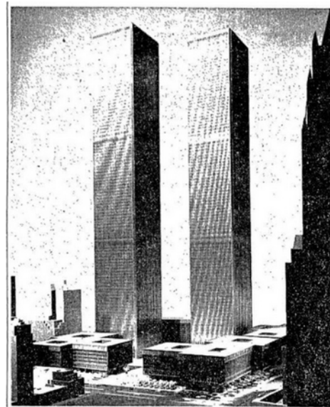
New Yorkin maailmankaupan keskus on valmistuttuun maailman korkein rakennus, josta kaksi 110-kerroksista tornia kohoavat yli 400 metrin korkeuteen. Rakennuskompleksi valmistuu tänä vuonna.
